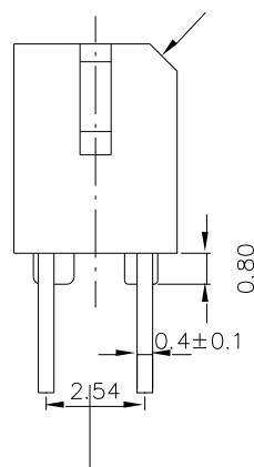
A-A' Section
